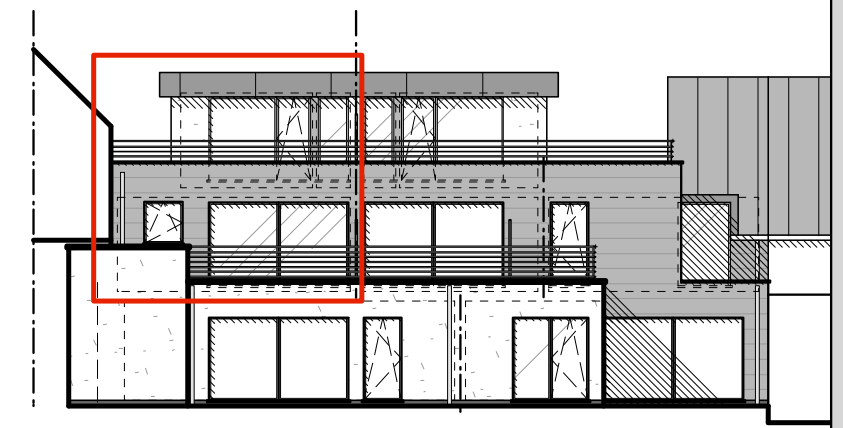
achtergevel 1/50
