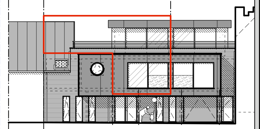
voorgevel 1/50
