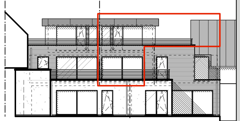
achtergevel 1/50
