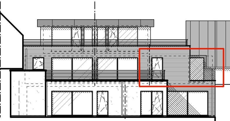
achtergevel 1/50
